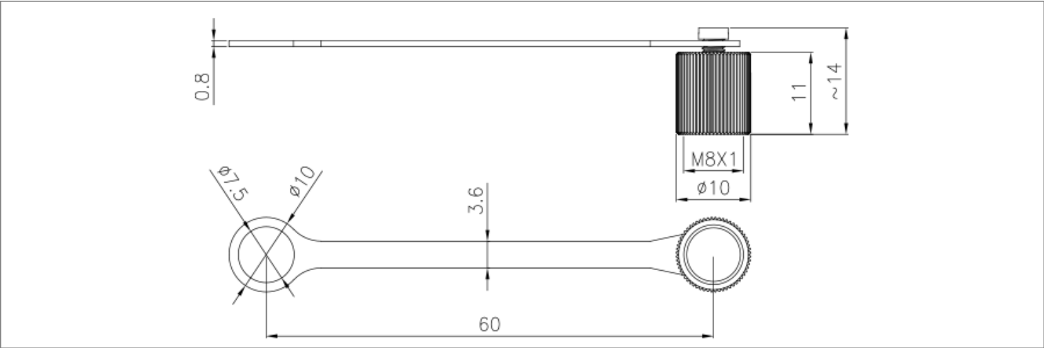
尺寸图
