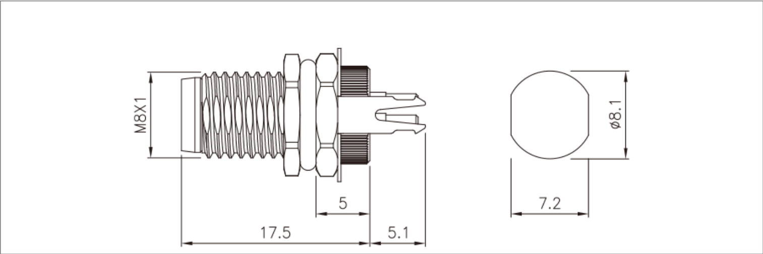
PCB直式芯位图(接地款)
