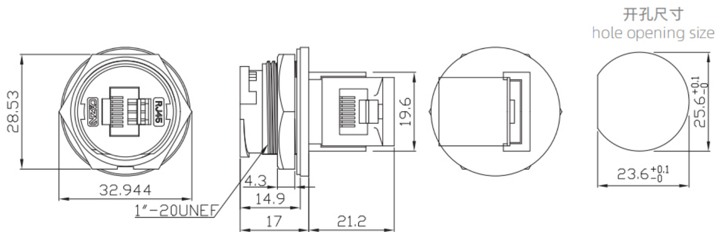
尺寸图
