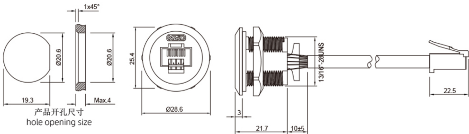
尺寸图
