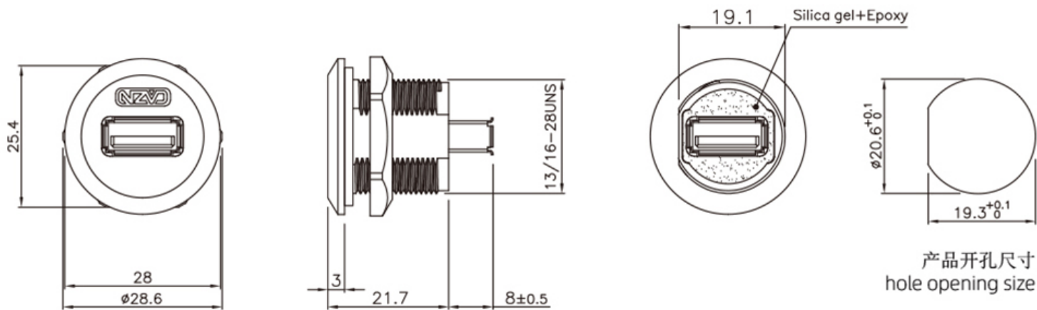
尺寸图
