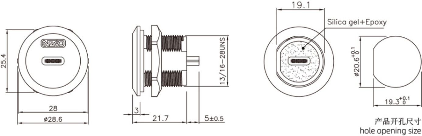
尺寸图
