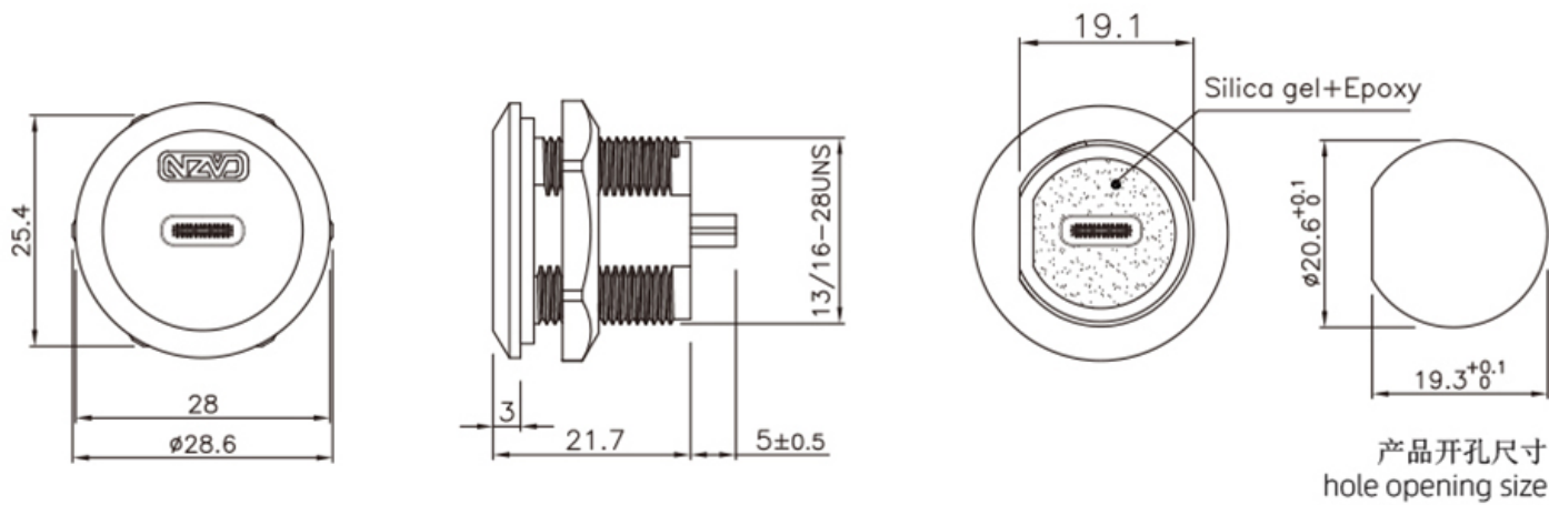
尺寸图
