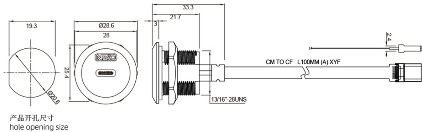
尺寸图
